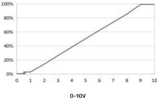
Curva de dimerización
